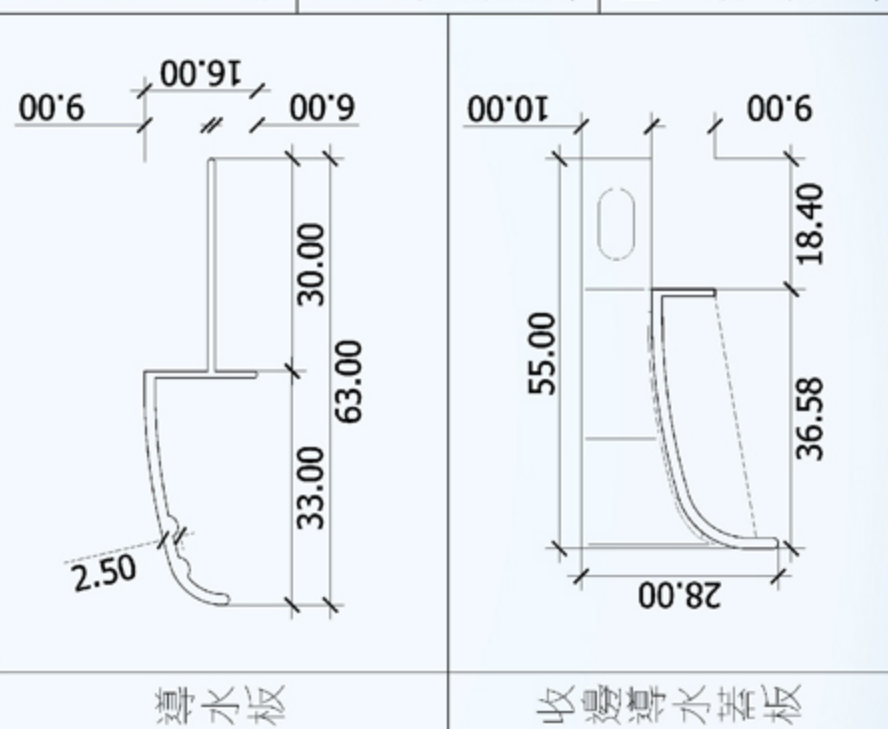
導水板施作大樣詳圖
